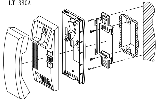
安裝示意圖 LT-380A
