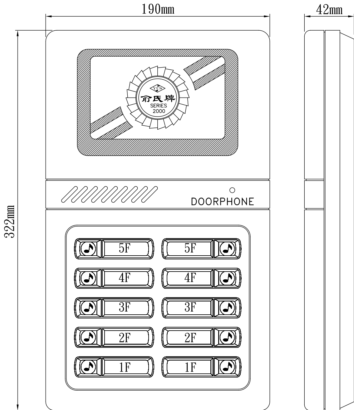
CD-03B-10 數位傳統型門口機
