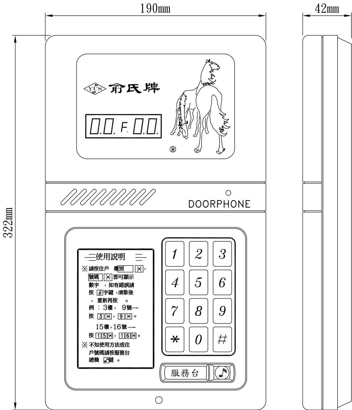
CD-2301ACS 數位顯示型門口機
