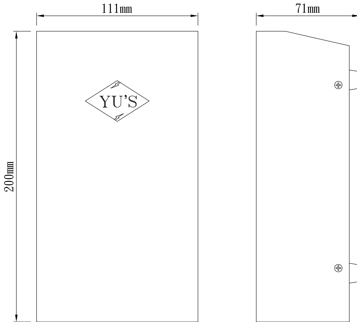
CP-2301A 數位電源主裝置
