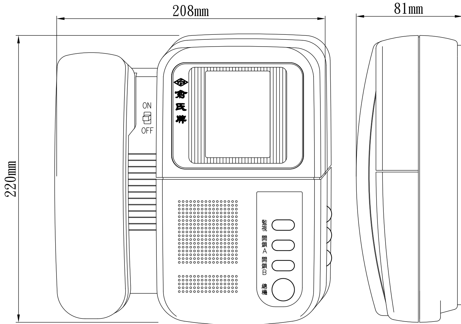
CR-02FCP 數位豪華型彩色影像室內機
