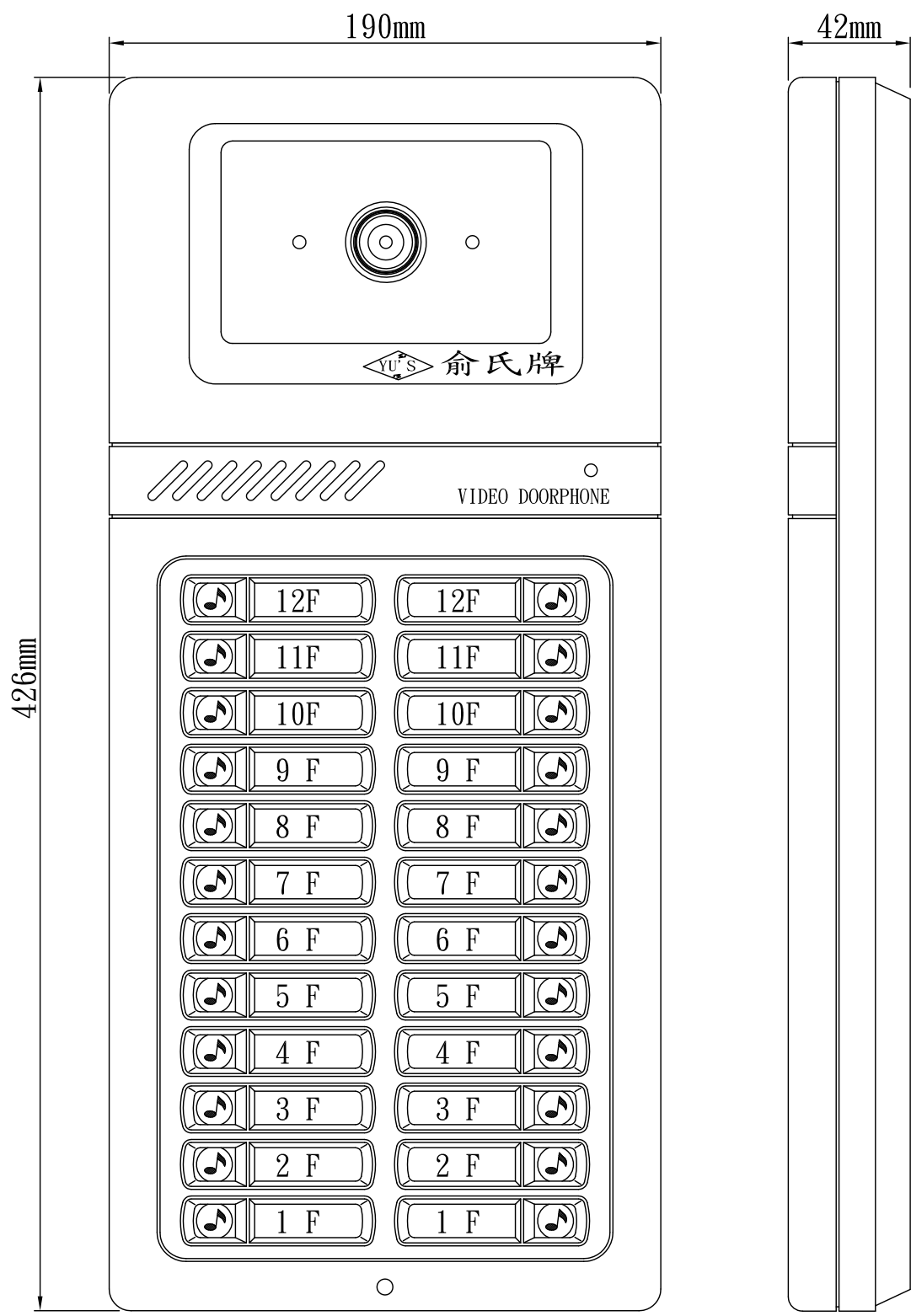
CV-23BC-24 數位傳統型彩色攝影門口機
