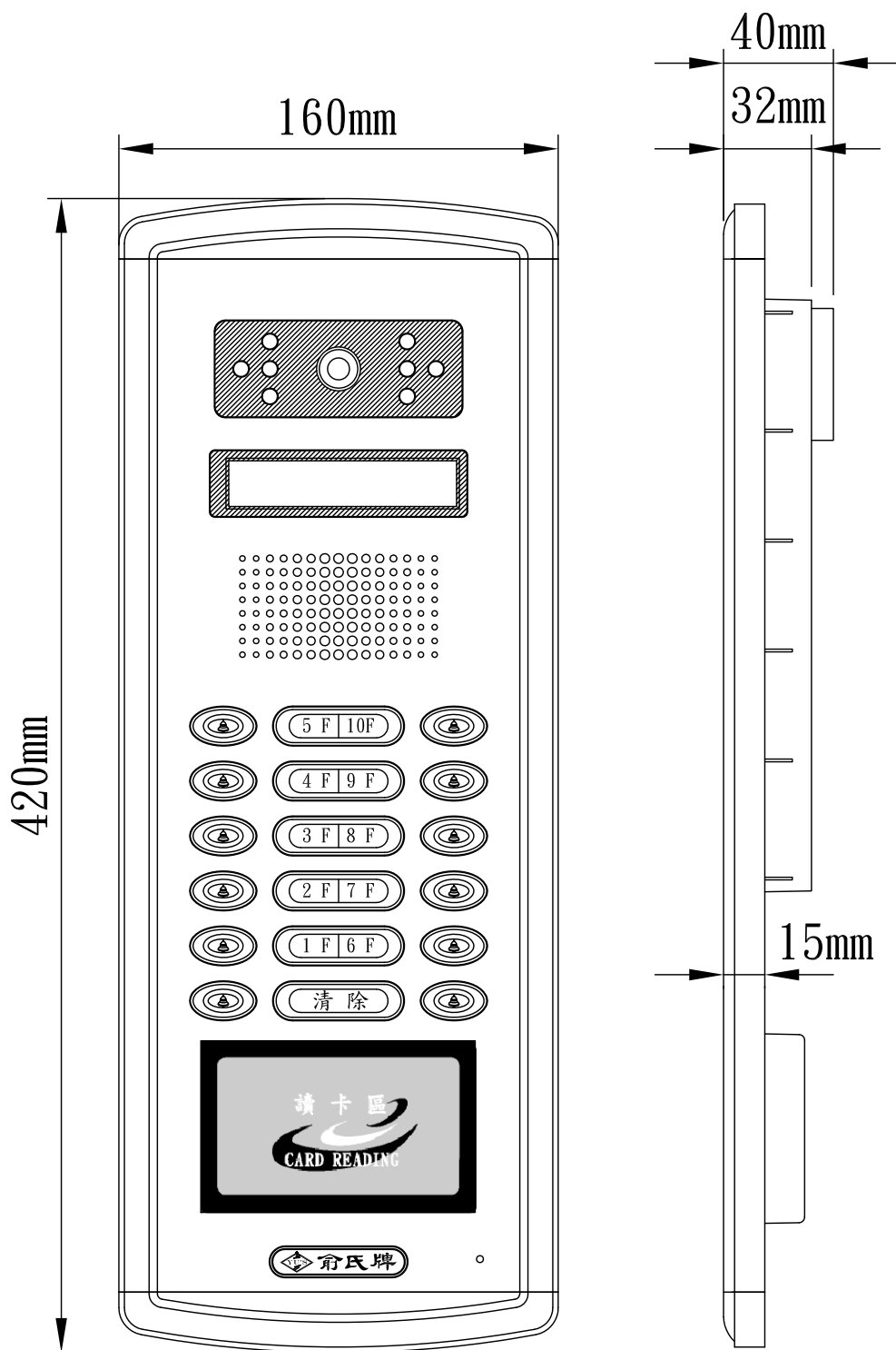
DFC3-10M2 嵌入式彩色攝影門口機 (含感應讀卡開鎖)
