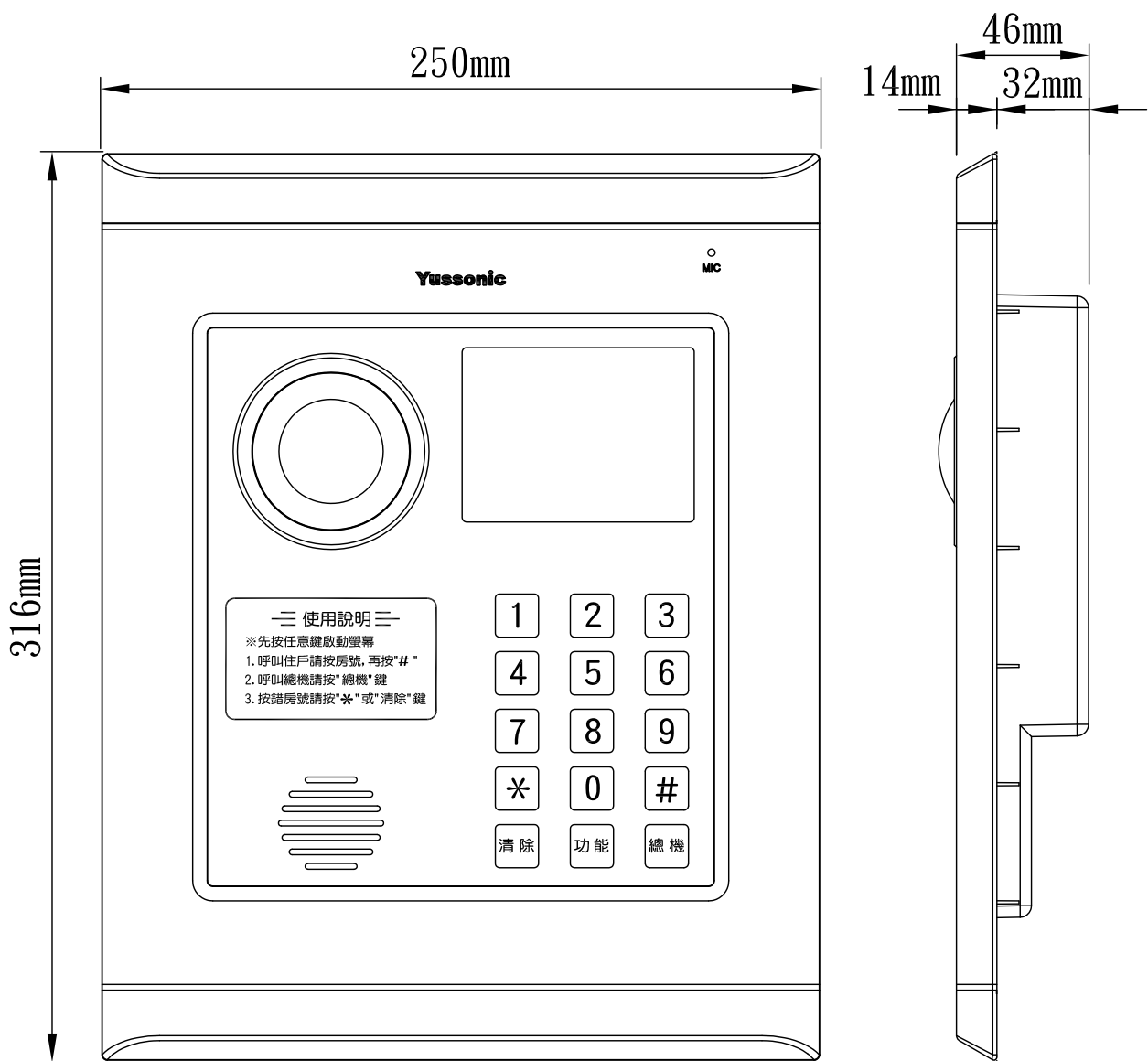
DHC2 嵌入式彩色攝影門口機 (含感應讀卡開鎖及語音導引)
