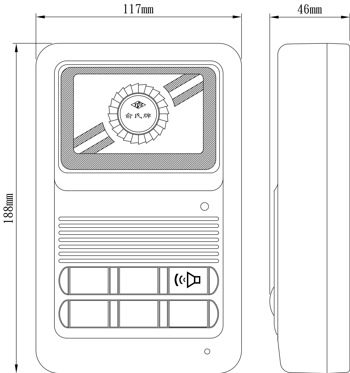
DP-265A-1 二線式單戶門口機
