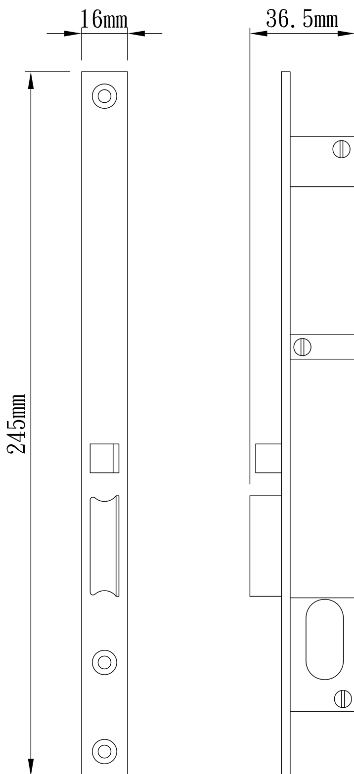
EL-203A-2 進口鋁門鎖2號
