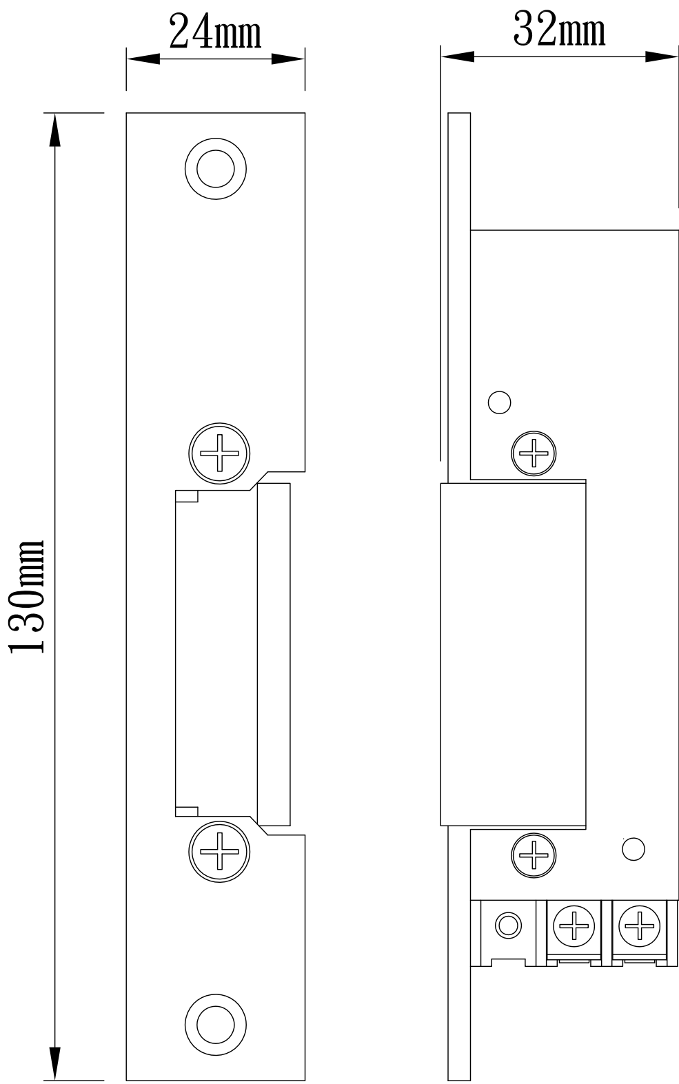
EL-209A 陰極鎖
