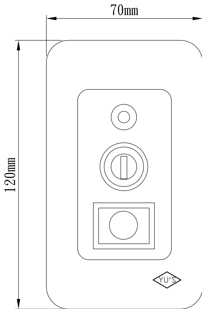
KS-02A 防盜控制鎖含門鈴按鈕
