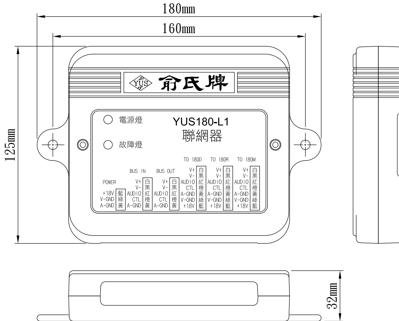
L1 聯網器
