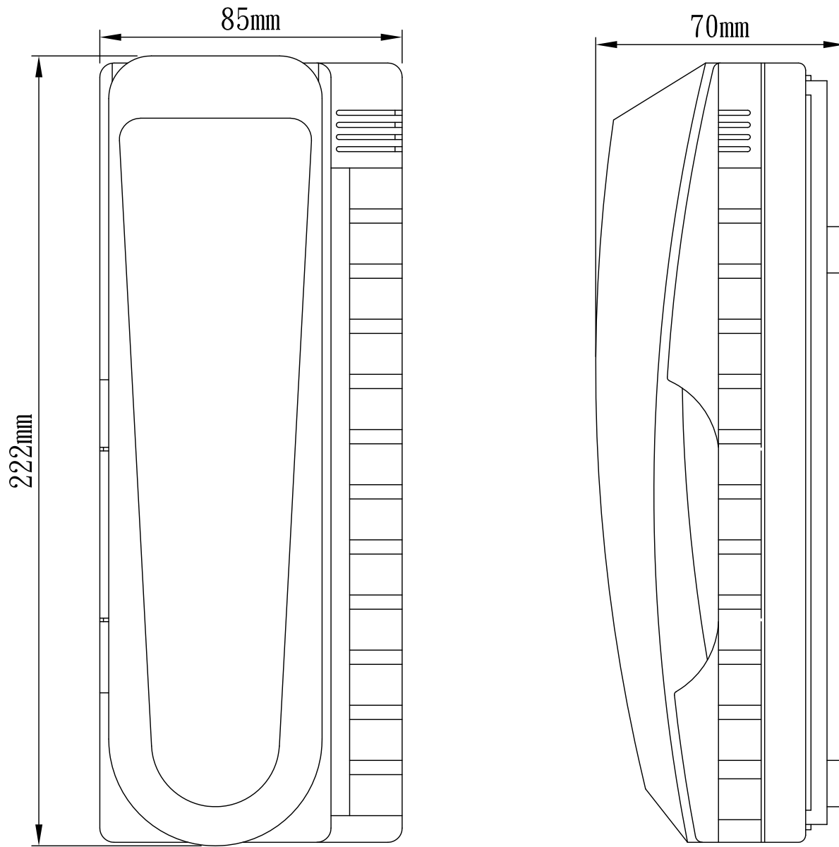
LT-101A 電梯分機(單局)
