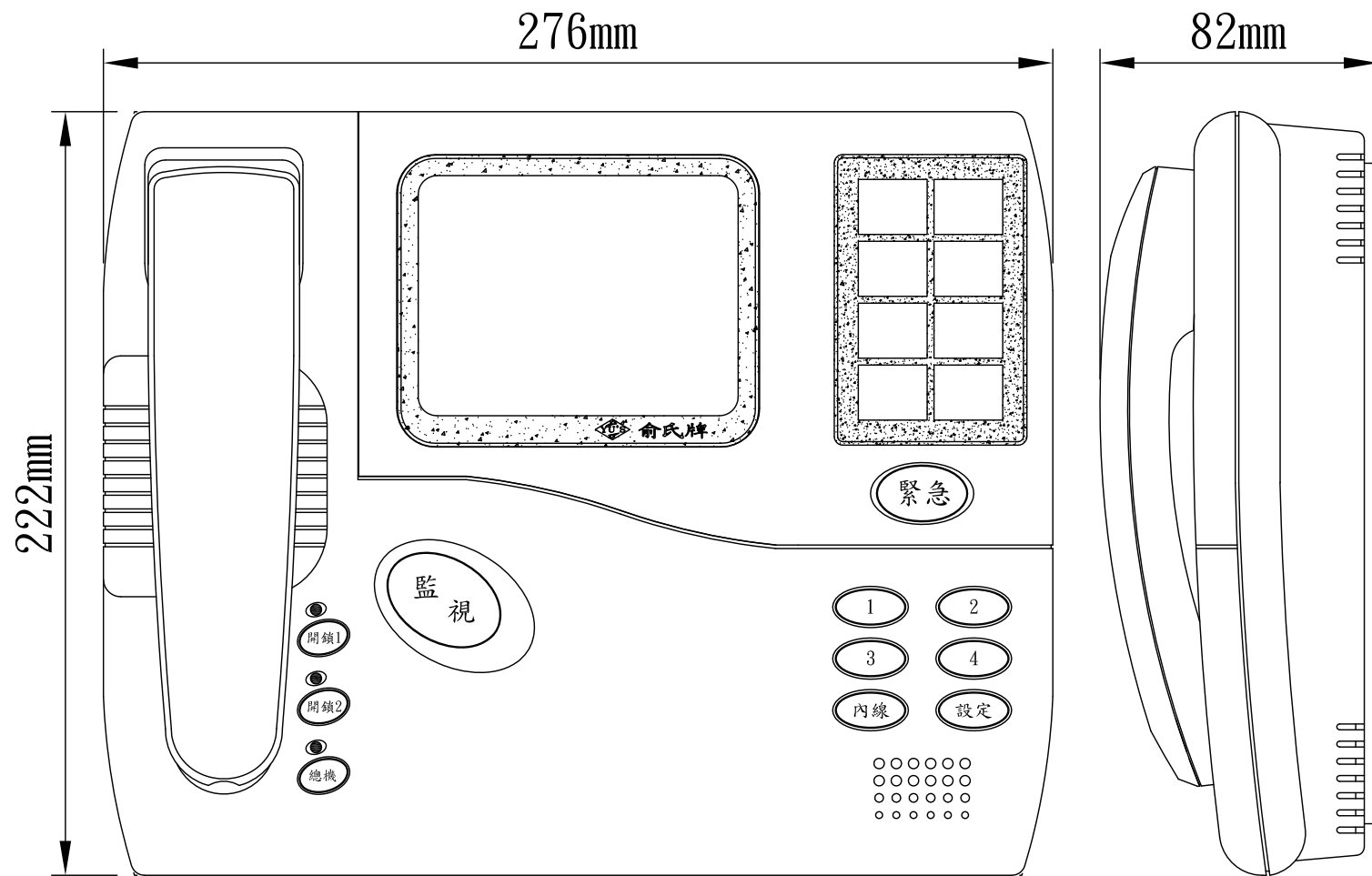
RBSC 防盜彩色影像室內機
