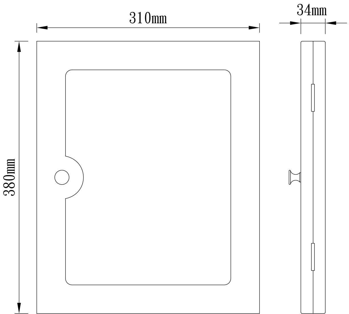
DH 防雨箱(右開型)
