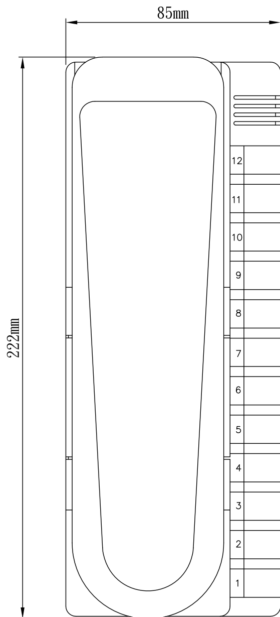
TU-12F 室內對講機
