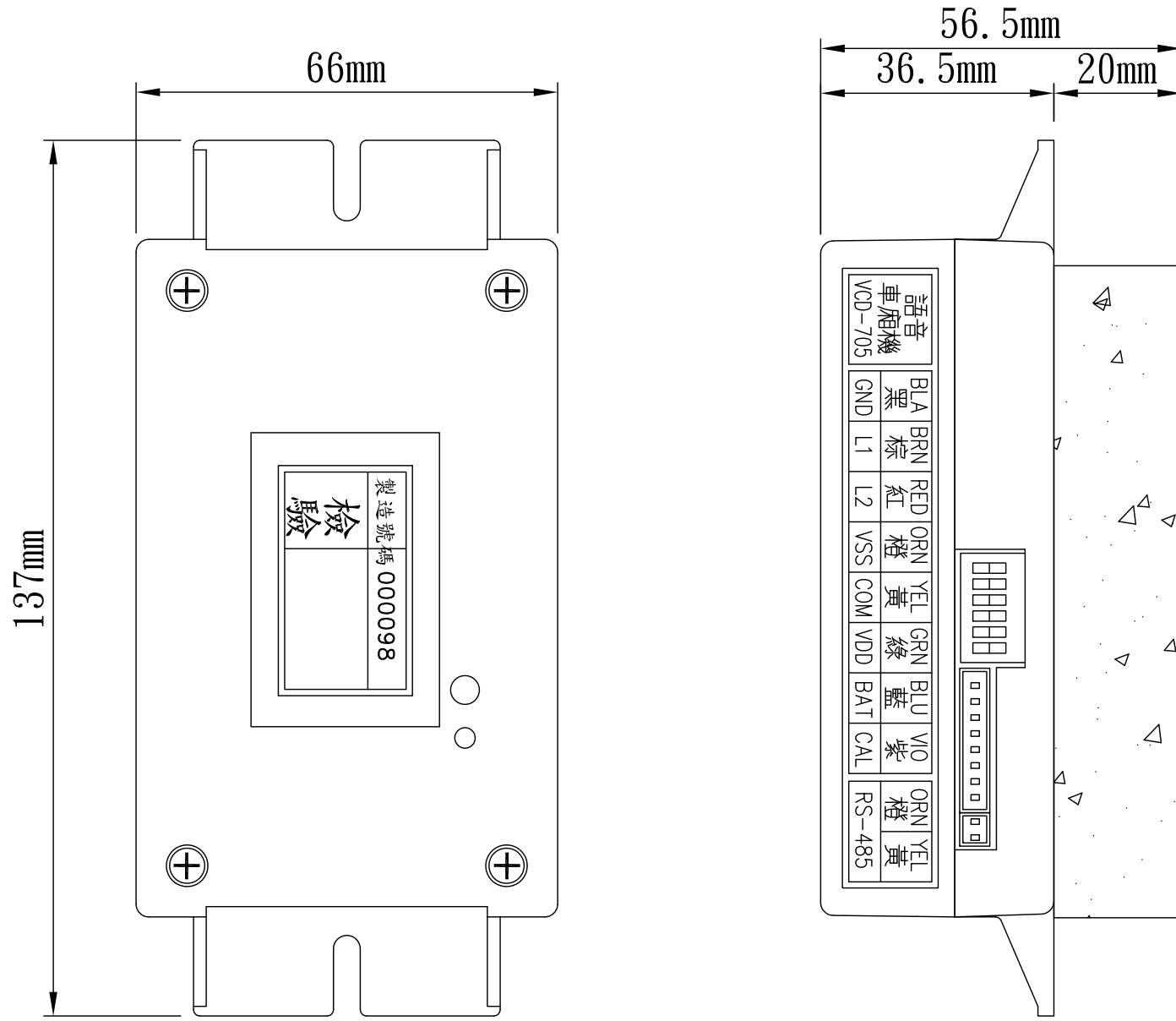
VCD-705 數位電梯語音車廂機
