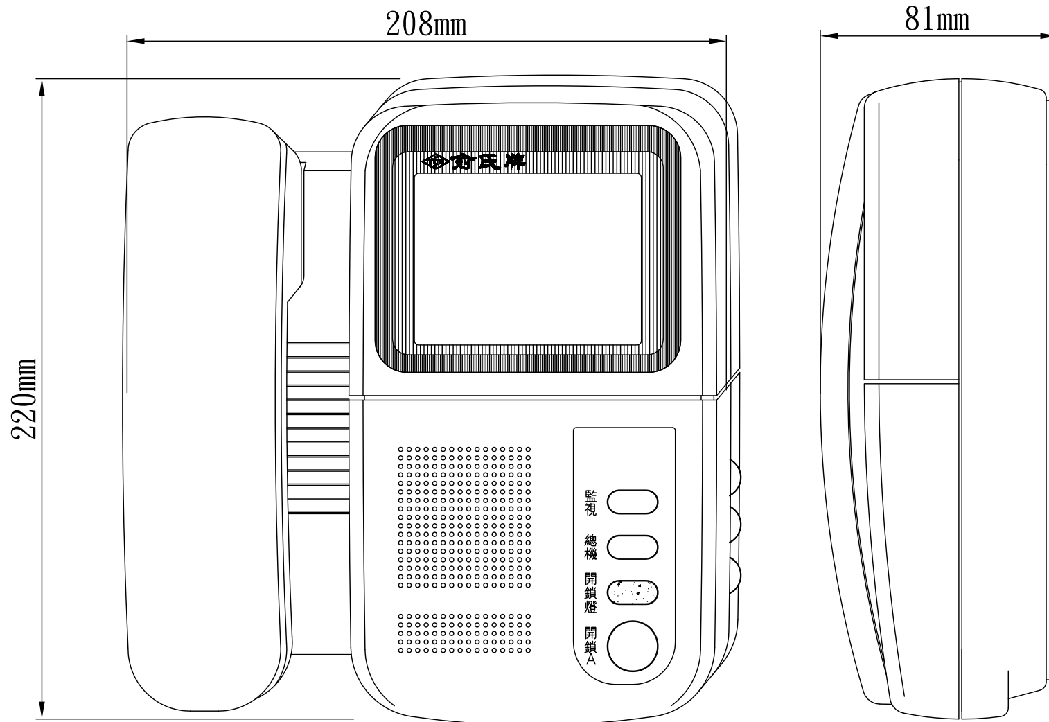
VR-02DC 超薄型彩色影像室內機
