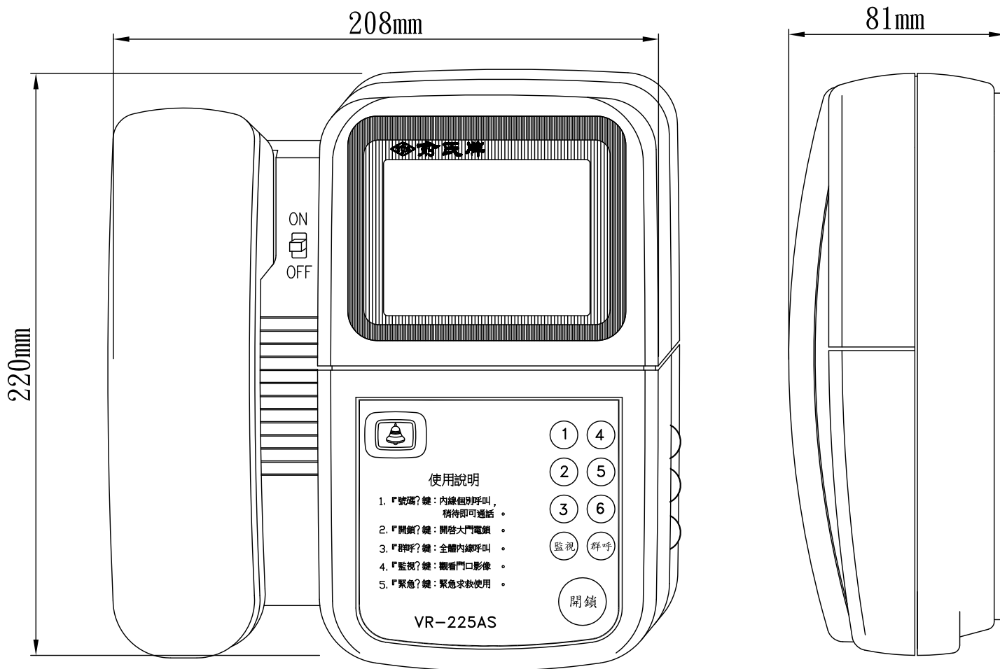
VR-225ASC 四線式六戶防盜彩色影像室內機
