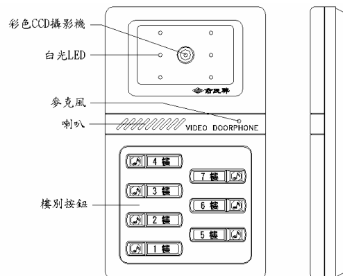
VD-275AC-7 四線式七戶彩色攝影門口機
