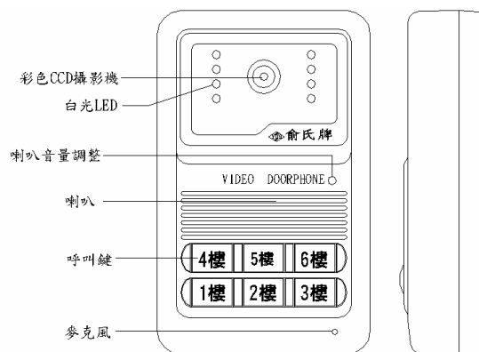
VD-265AC-6 四線式六戶彩色攝影門口機
