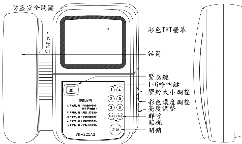
VR-225ASC 四線式六戶防盜彩色影像室內機
