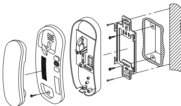
安裝示意圖
