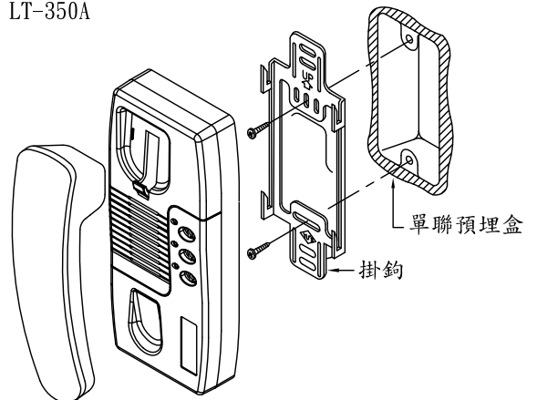
安裝示意圖 LT-350A
