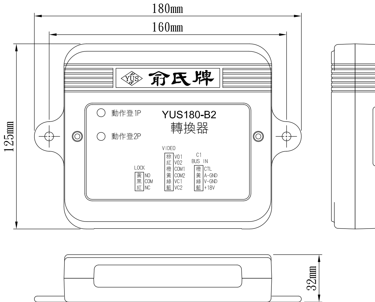
B2 轉換器
