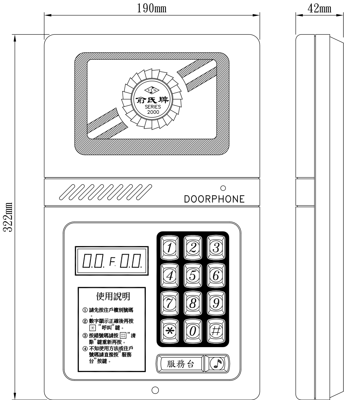
CD-01ACS 數位顯示型門口機
