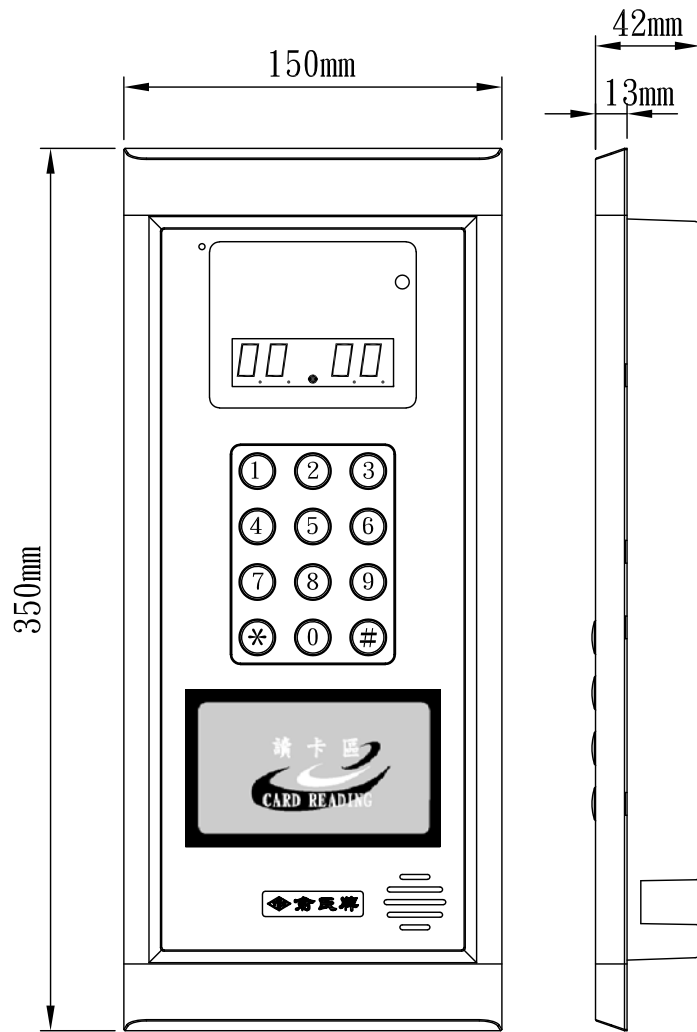
CD-108A 數位四線式門口機 (嵌入式)
