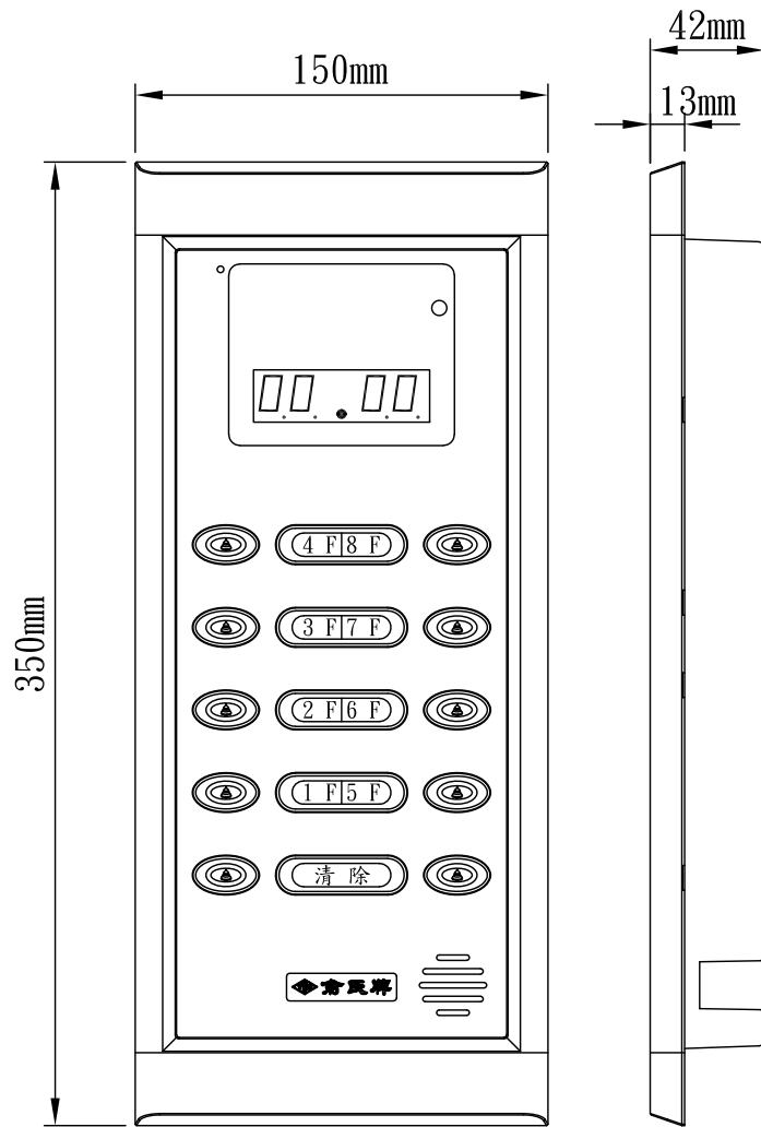
CD-108B-8 數位四線式影門口機 (嵌入式)
