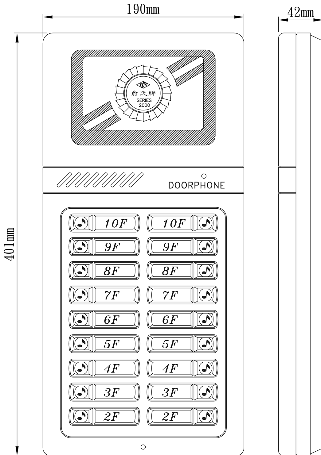
CD-13B-18 數位傳統型門口機
