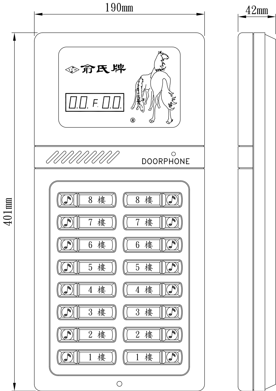
CD-2313B-16 數位顯示型門口機
