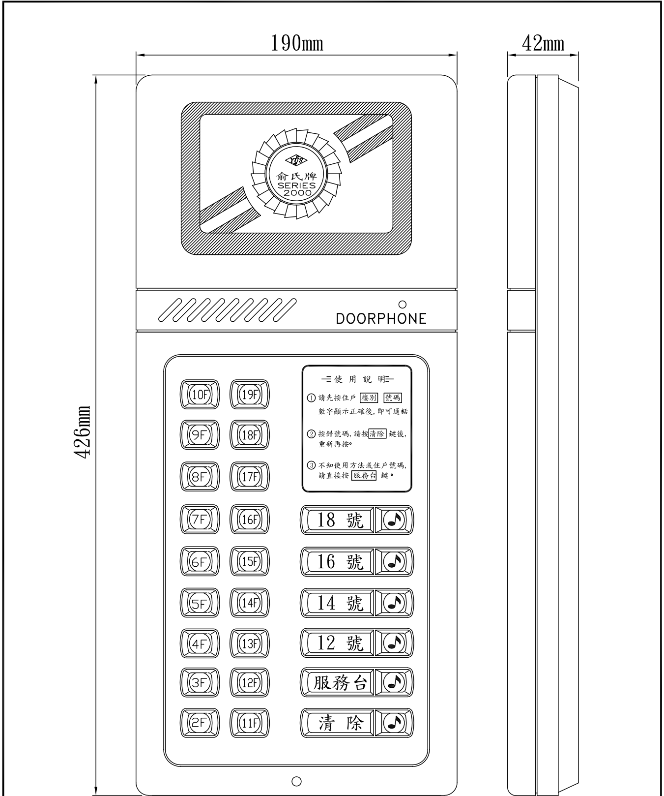
CD-29CCS-72 數位傳統型門口機
