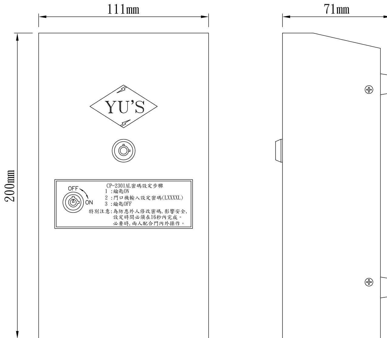
CP-2301AL 數位電源主裝置(密碼鎖)
