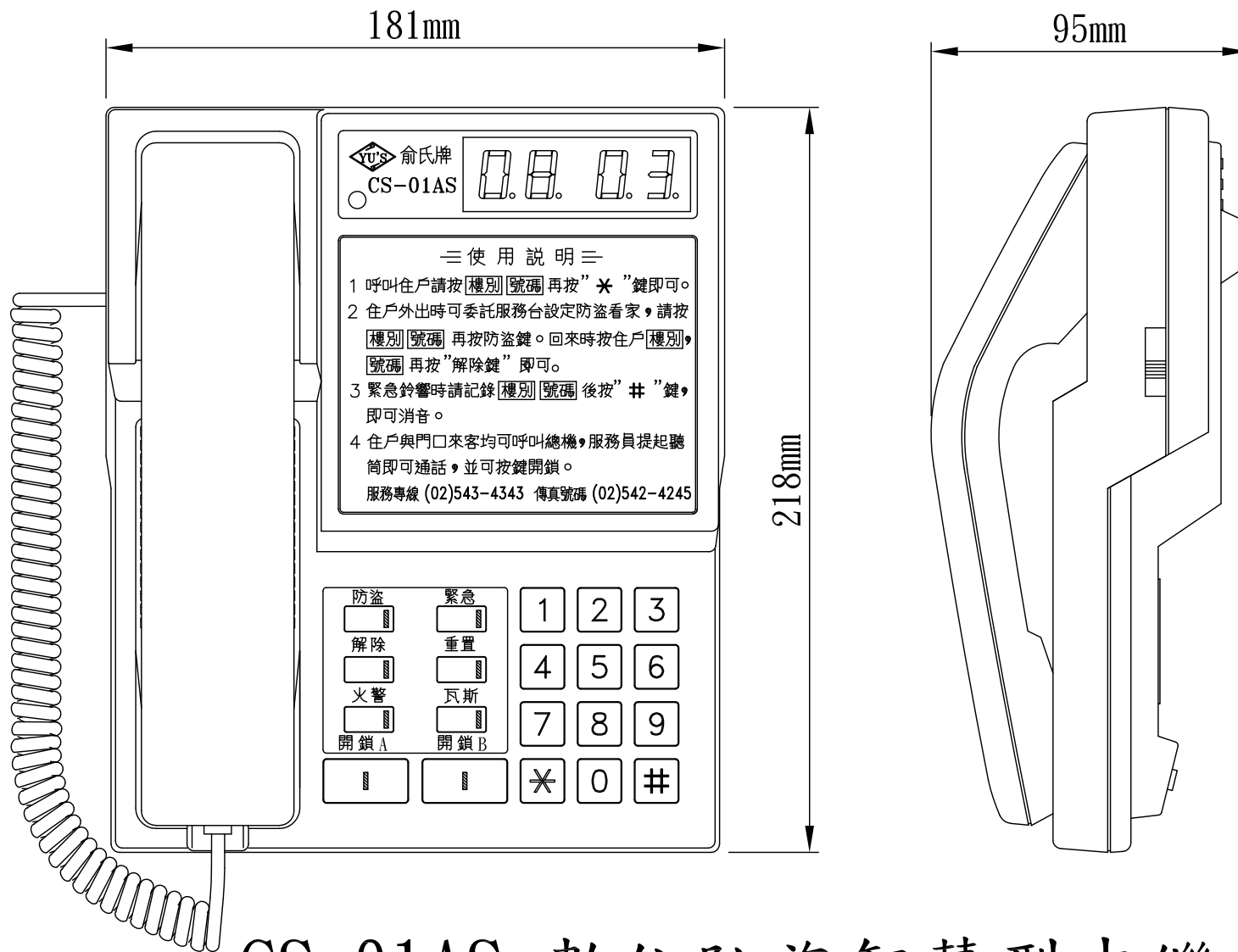
CS-01AS 數位防盜智慧型中繼台
