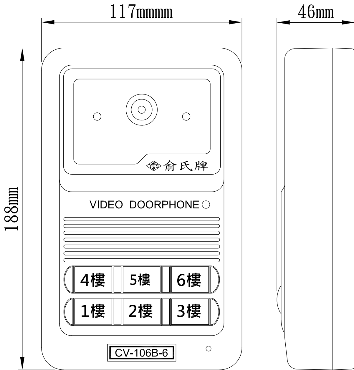
CV-106B-6 數位四線式彩色攝影門口機
