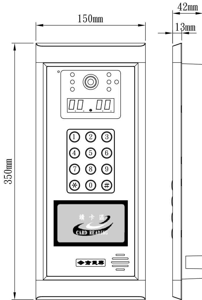
CV-108A 數位四線式彩色攝影門口機 (嵌入式)
