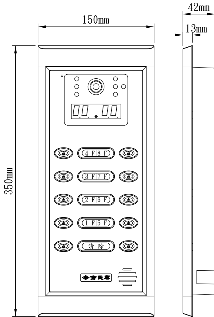
CV-108B-8 數位四線式彩色攝影門口機 (嵌入式)
