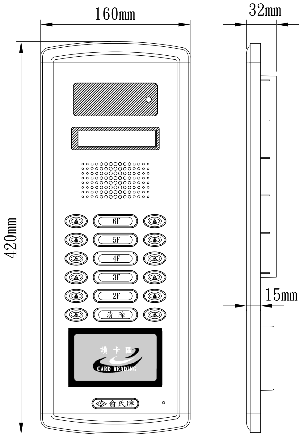
DFN3-10M2 嵌入式門口機 (含感應讀卡開鎖)
