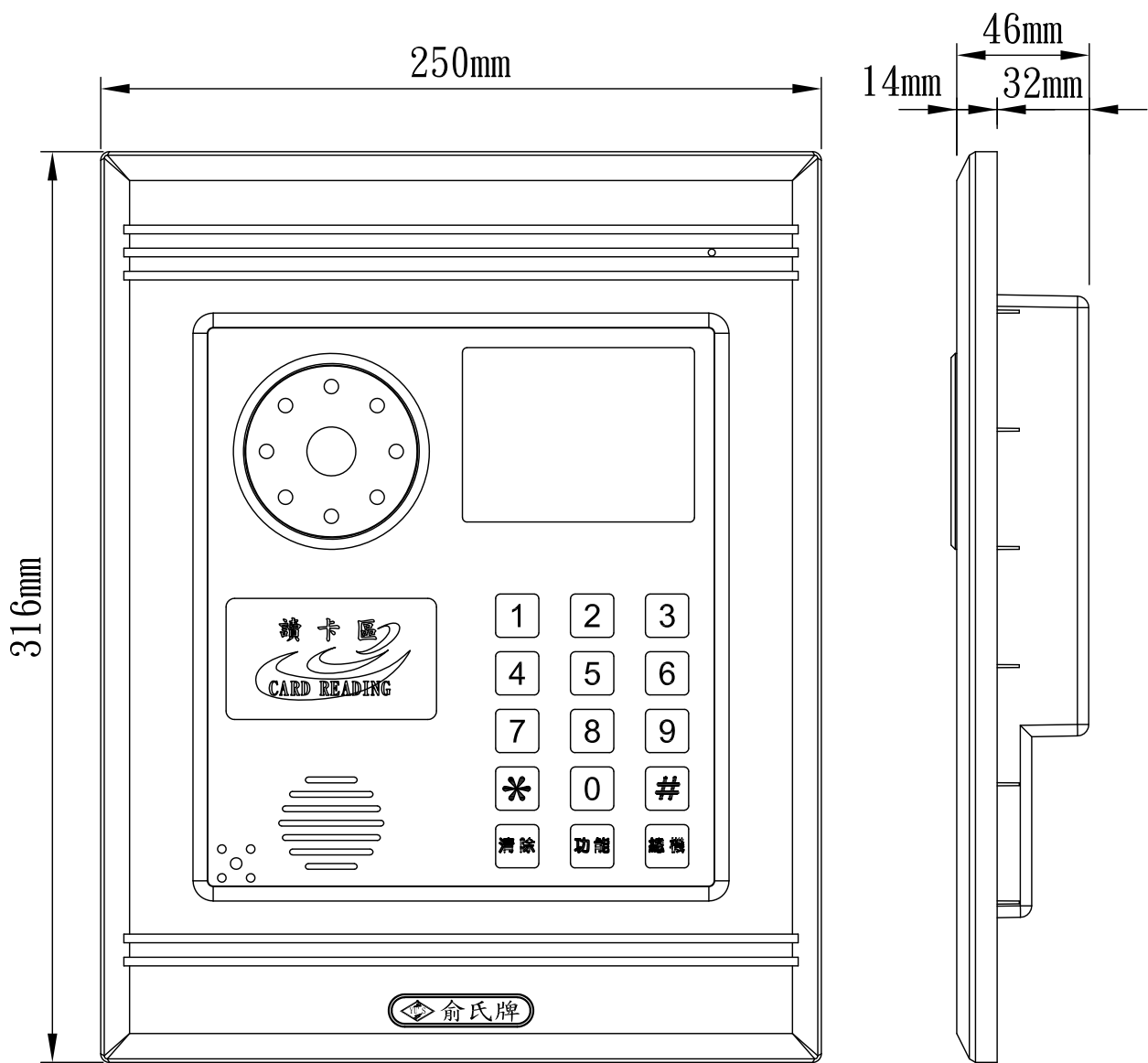
DHA1 嵌入式彩色攝影門口機 (含感應讀卡開鎖及語音導引)
