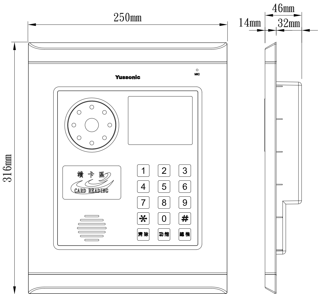
DHC1-M 嵌入式彩色攝影門口機 (含感應讀卡開鎖及語音導引)
