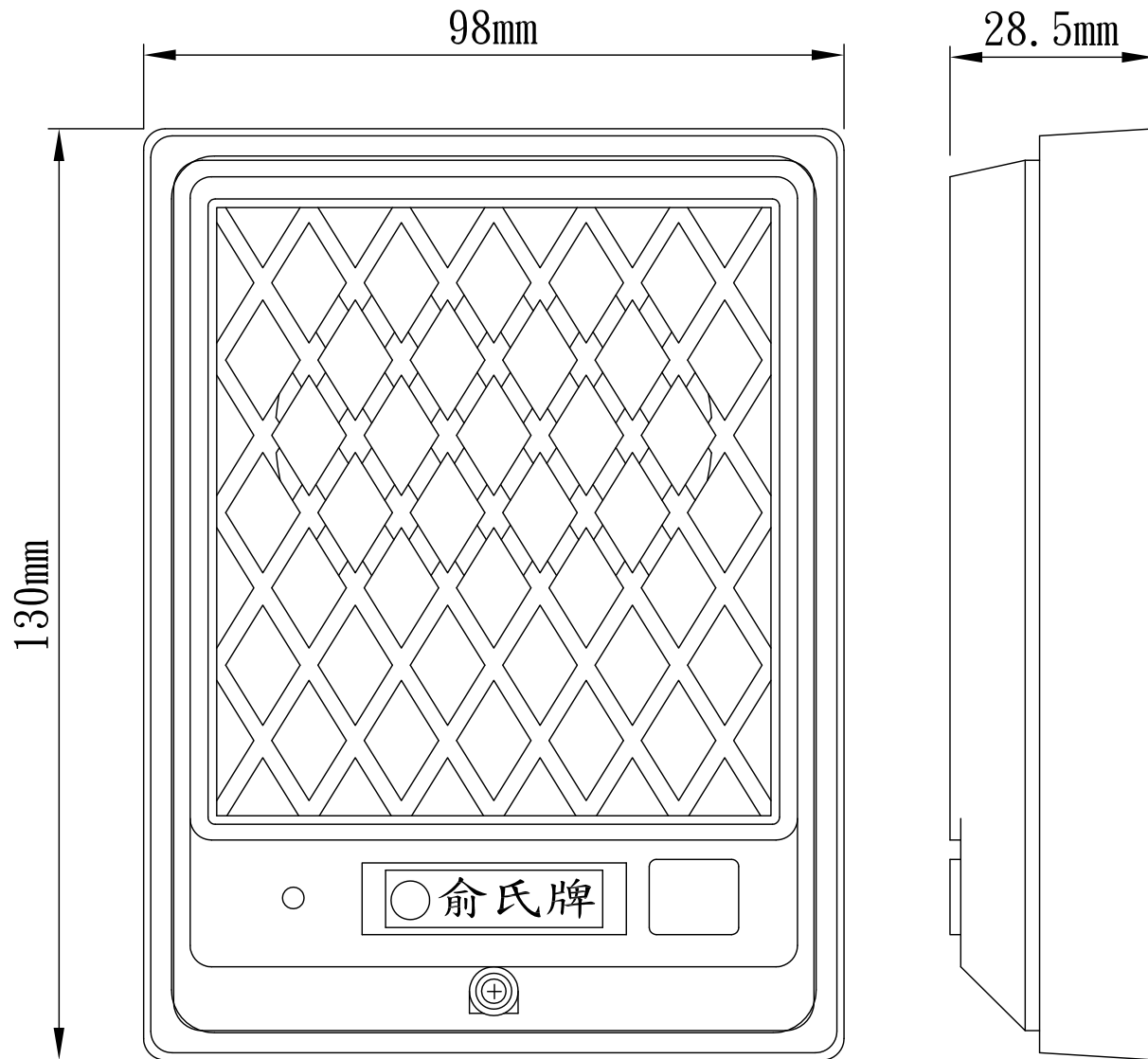
DP-10A 單戶門口機
