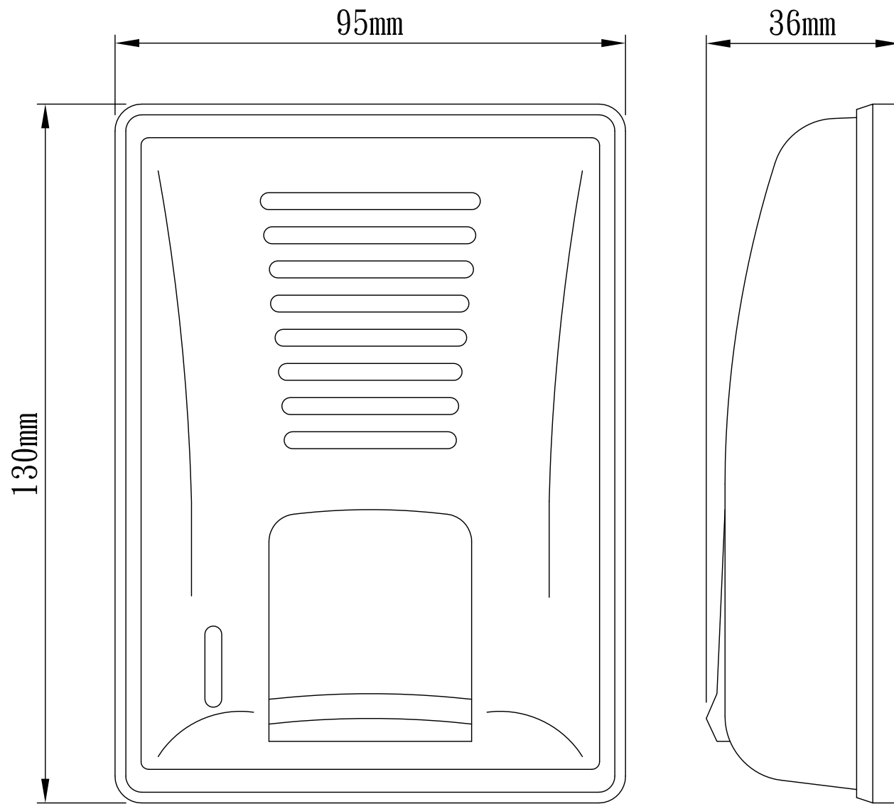
DP-12B 二線式門口機
