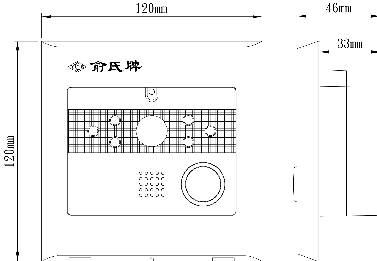
DVC2-1 嵌入式彩色攝影玄關機
