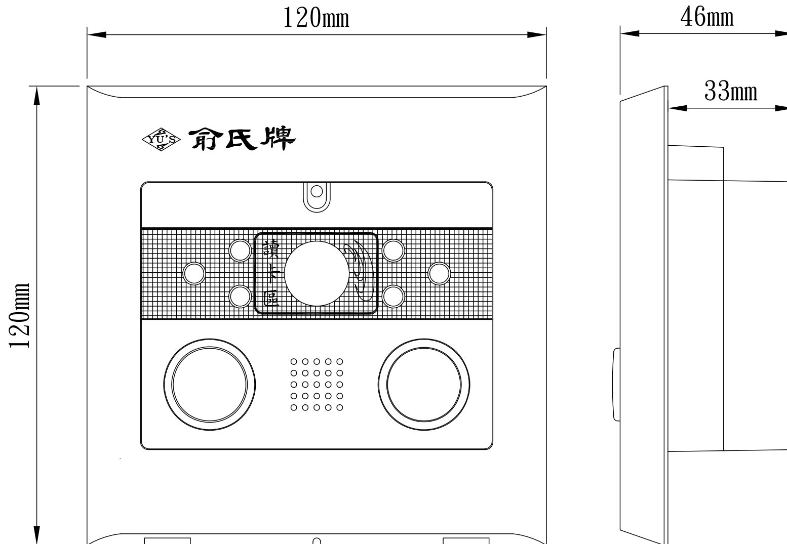
DVC2-1M 嵌入式彩色攝影玄關機 (含讀卡設定外控鎖)
