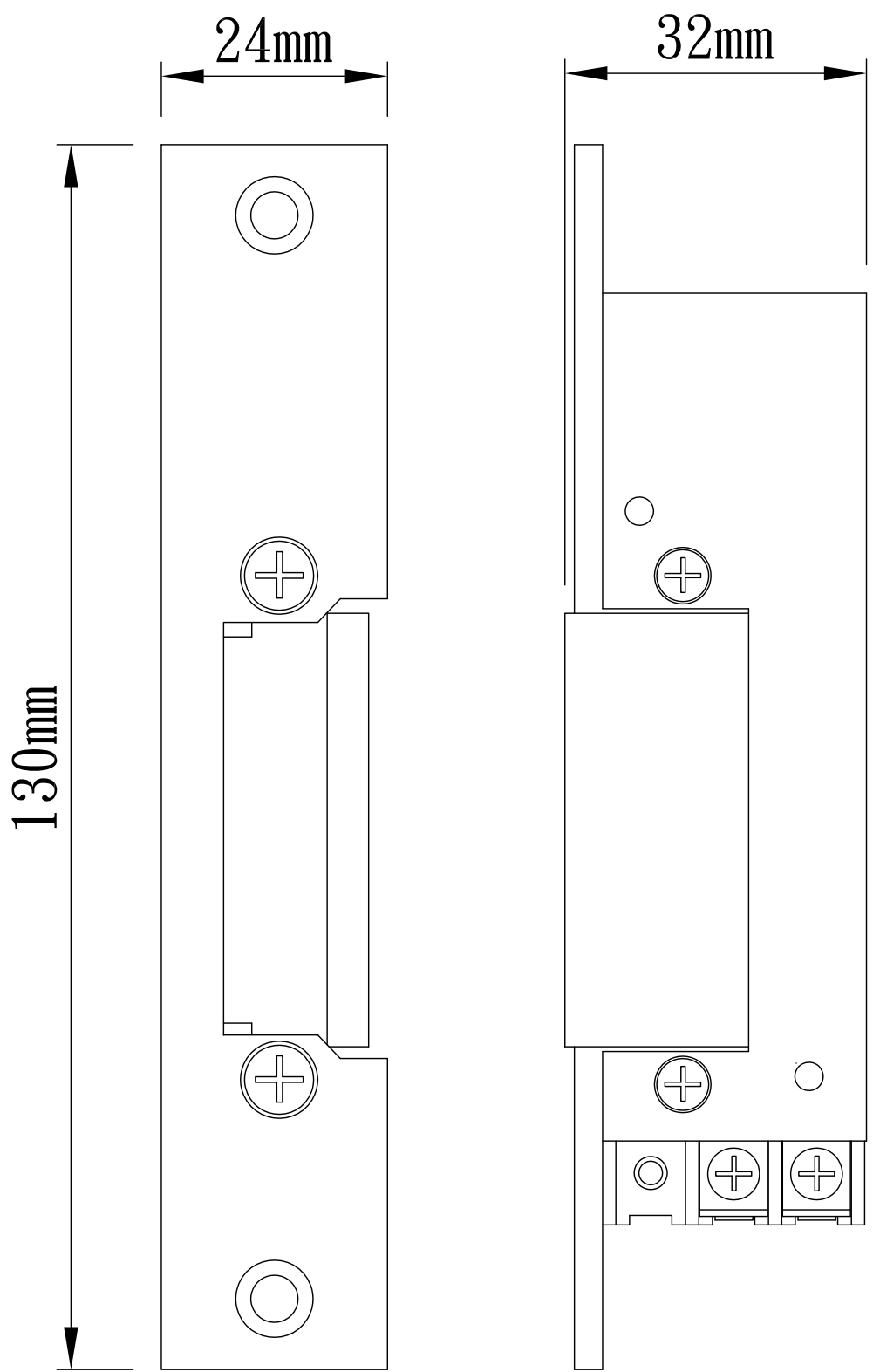
EL-209B 自動式陰極鎖
