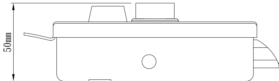
EL-371L 可鎖式電鎖(外開)
