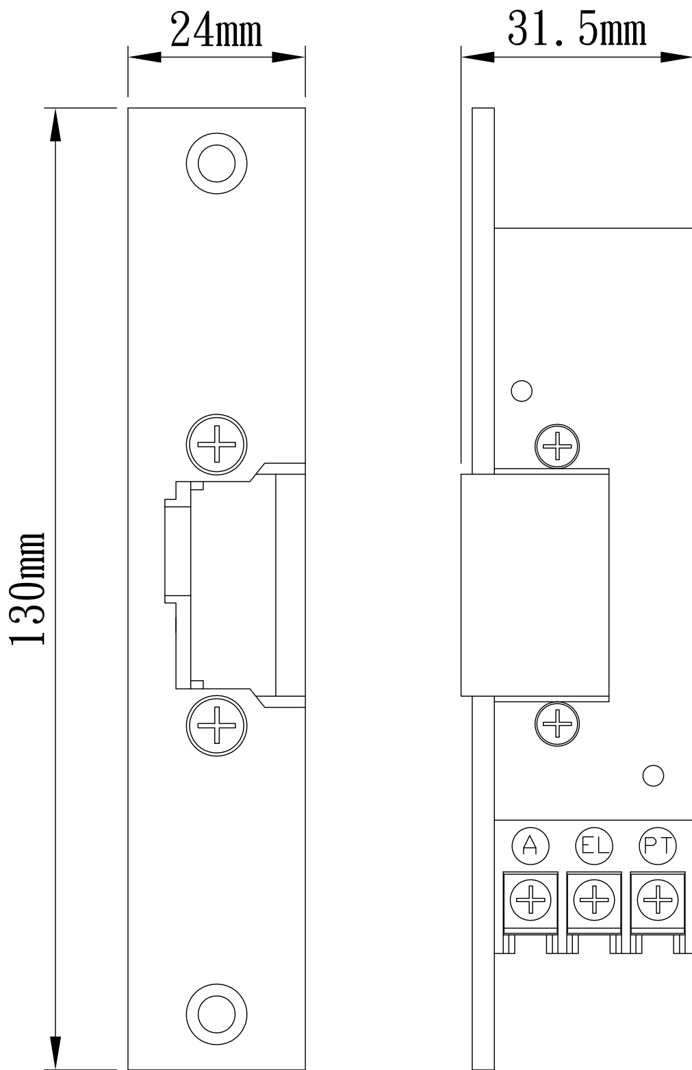
EL-391A 陰極鎖
