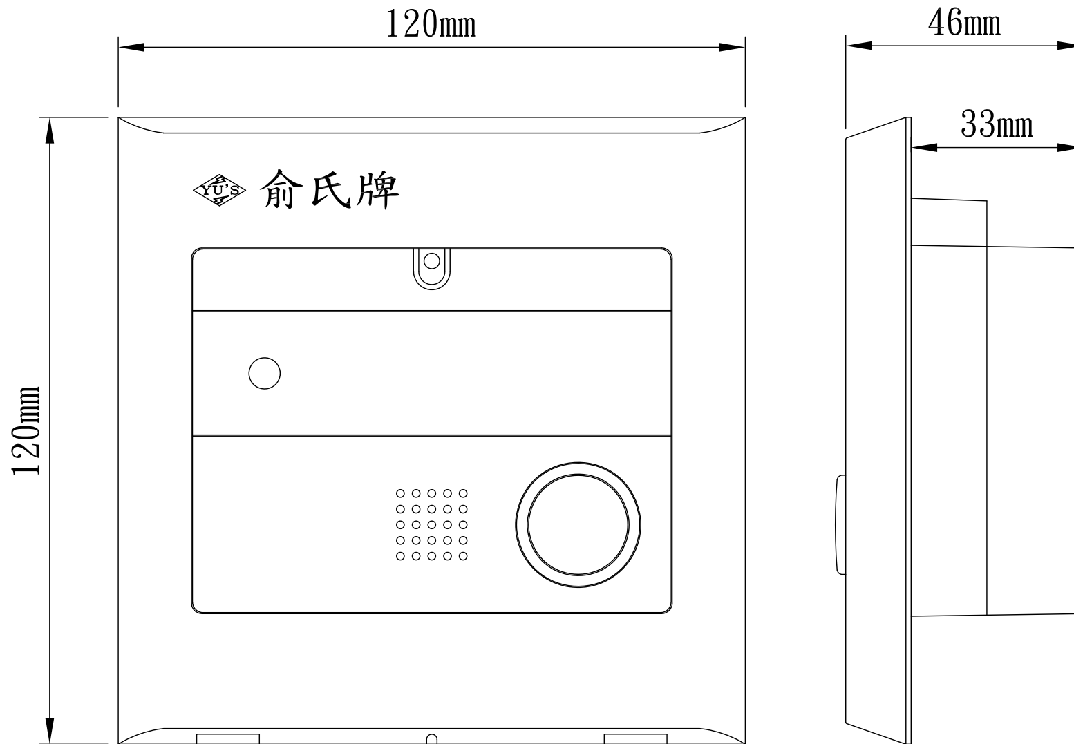
EN3 嵌入式緊急對講機
