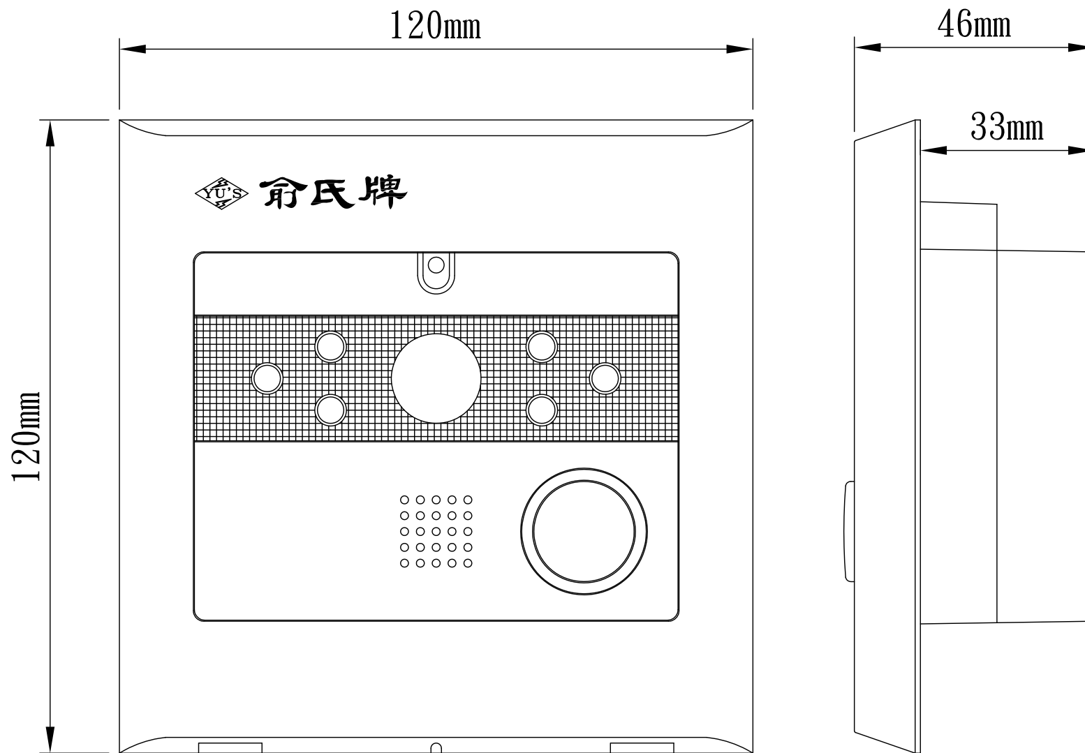
EVC3 嵌入式彩色攝影緊急對講機
