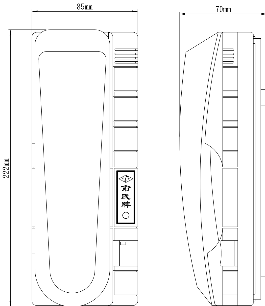
LT-190BL 二線式可開鎖室內機
