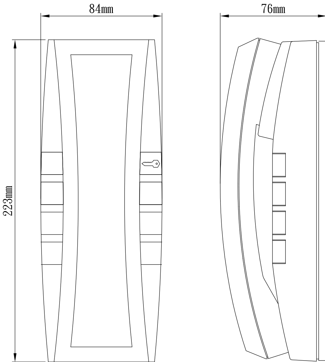
LT-385B 室內機(室內兼門口對講)
