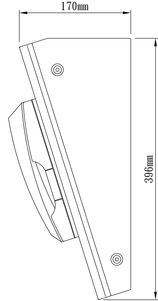
MB-410AC 電梯總機(訂製品)
