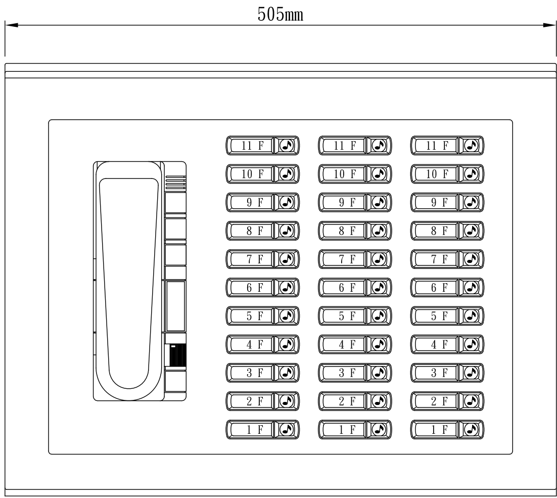
MB-410AC 電梯總機(訂製品)
